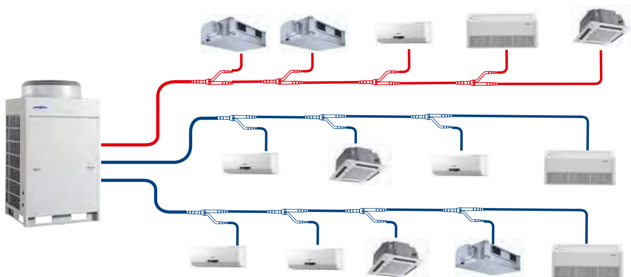
Пример установки с 3 трубами
